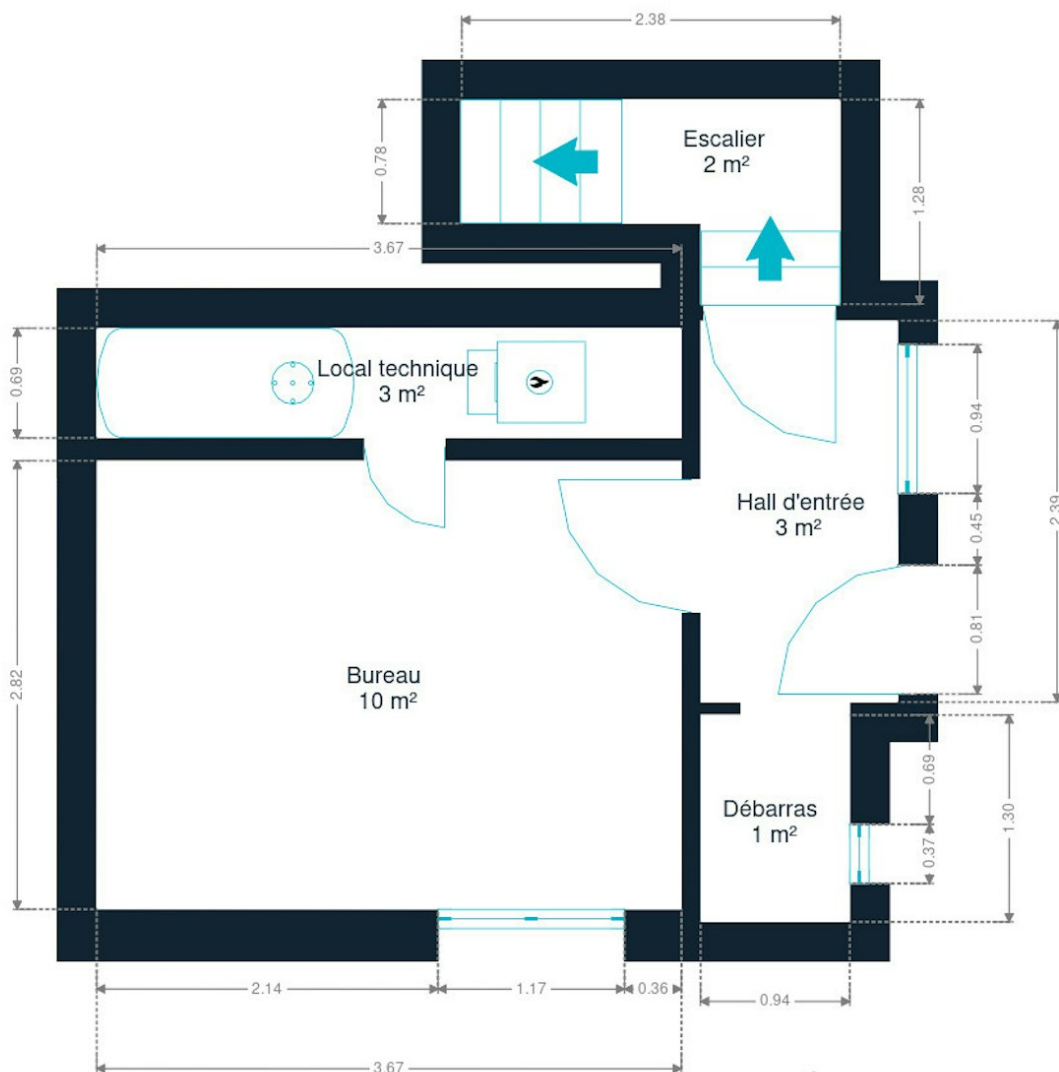
Rez-de-chaussée
